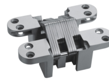
型号: HCG002 尺寸: 28X118X22mm
