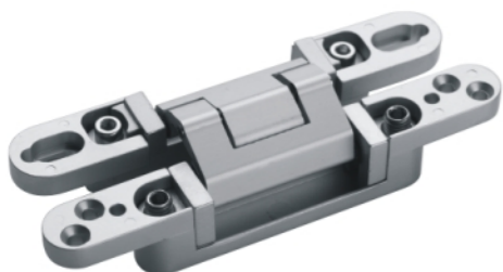
型号: HBG007 (不分左右) 尺寸: 140x135x18x21x23mm
