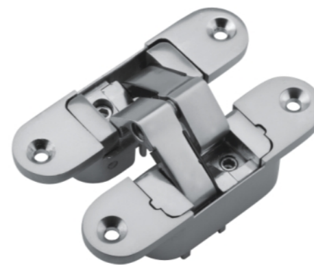
型号: HBG001 (左开式) HBG002 (右开式) 尺寸: 30X110mm (可以订做不锈钢精铸摇臂)
