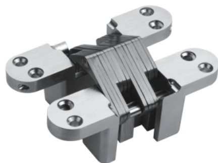
型号: HAG002 尺寸: 28X118X22mm
