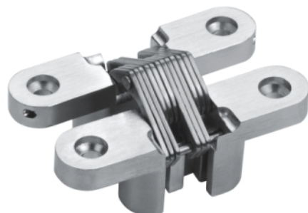
型号: HAG005 尺寸: 16X70X11mm
