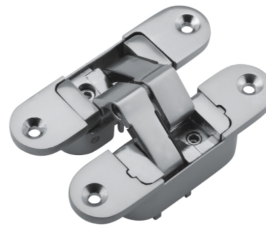
型号: HBG001 (左开式) HBG002 (右开式) 尺寸: 30X110mm
