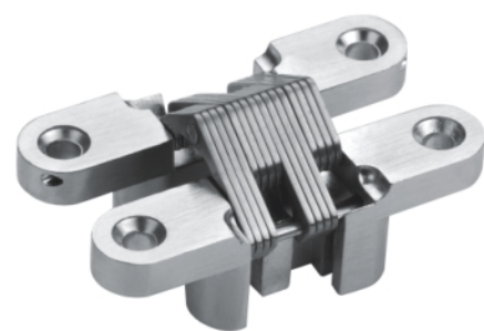
型号: HAG006 尺寸: 13X60X9mm
