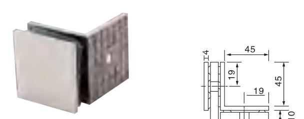
GC-009 方形固定夹90° 单面 Square fixing clip 90° Single
