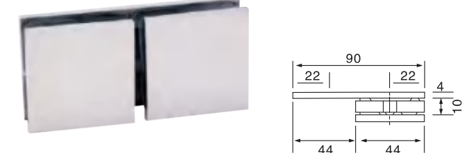
GC-011 方形固定夹180° 双面 Square fixing clip 180° Double
