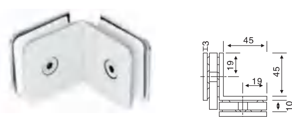
GC-002 方形固定夹90° 双面 Square fixing clip 90° Double
