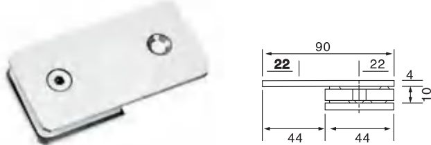
GC-004 方形固定夹180° 单面 Square fixing clip 180° Single
