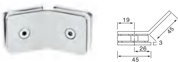
GC-003 方形固定夹135° 双面 Square fixing clip 135° Double
