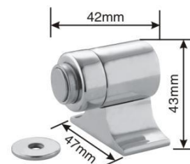
型号: HDS026(锌合金) 尺寸: 47 \times 42 \times 43 \text{mm}
