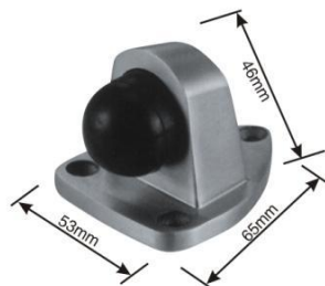
型号: HDS058(不锈钢精铸) 尺寸: 65 \times 53 \times 46 \text{mm}
