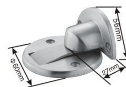
型号: HDS048(不锈钢精铸) 尺寸: \Phi 60X56mm
