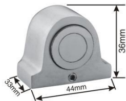
型号: HDS051(不锈钢精铸) 尺寸: 44 \times 33 \times 36 \text{mm}
