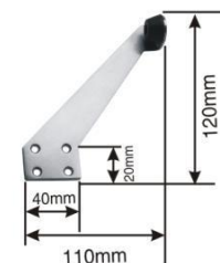
型号: HDS073右门顶(不锈钢冲压) 尺寸: 40 \times 110 \times 120 \text{mm}
