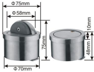
型号: HDS075 隐形门顶(不锈钢精铸) 尺寸: \Phi 75 \times 75 \text{mm}
