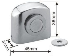
型号: HDS029(不锈钢精铸) 尺寸: 45X31X38mm
