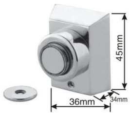
型号: HDS028(锌合金) 尺寸: 36X34X45mm
