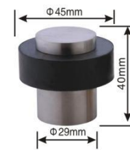
型号: HDS020B(锌合金) 尺寸: \Phi 29 \times 40 \text{mm}
