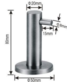
型号: HDS077(不锈钢) 尺寸: 50 \times 80 \text{mm}
