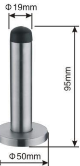
型号: HDS081(不锈钢) 尺寸: \Phi 50 \times 95 \text{mm}
