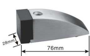
型号: HDS037(不锈钢精铸) 尺寸: 76X28X28mm
