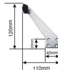
型号: HDS072左门顶(不锈钢冲压) 尺寸: 40 \times 110 \times 120 \text{mm}
