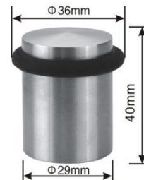
型号: HDS043(不锈钢) 尺寸: \Phi 29X40mm
