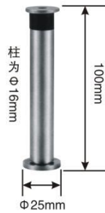
型号: HDS083(不锈钢门吸) 尺寸: 25 \times 100 \text{mm}
