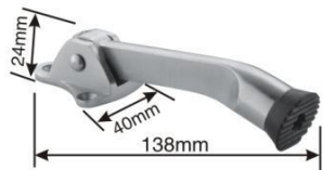
型号: HDS032(锌合金) 尺寸: 138X40X24mm
