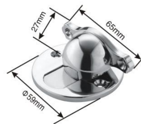
型号: HDS045(锌合金) 尺寸: \Phi 59X65mm
