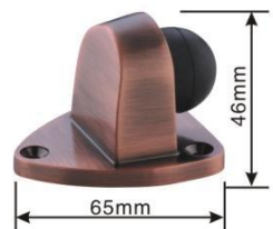
型号: HDS031(锌合金) 尺寸: 65X52X46mm
