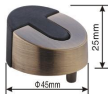
型号: HDS012(锌合金) 尺寸: \Phi 45 \times 25 \text{mm}
