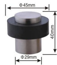
型号: HDS020(不锈钢) 尺寸: \Phi 29 \times 40 \text{mm}
