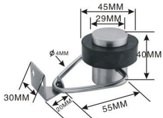
型号: HDS078(不锈钢) 尺寸: \Phi 29 \times 40 \times 45 \text{mm}
