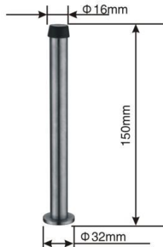
型号: HDS082(不锈钢实心棒加工) 尺寸: \Phi 32 \times 150 \text{mm}
