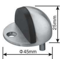
型号: HDS017B(不锈钢精铸) 尺寸: \Phi 45 \times 25 \text{mm}
