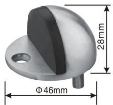
型号: HDS017(不锈钢精铸) 尺寸: \Phi 46 \times 28 \text{mm}
