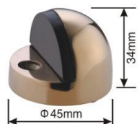
型号: HDS038(不锈钢精铸) 尺寸: \Phi 45X34mm
