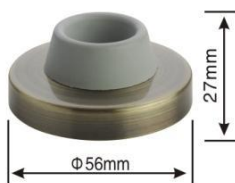
型号: HDS015(不锈钢) 尺寸: \Phi 56 \times 27 \text{mm}
